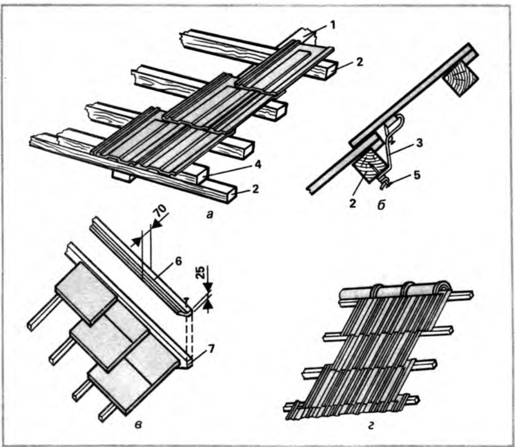
Рис. 12. Укладка пазовой ленточной черепицы: а — от карниза; б — закрепление на обрешетке; в — у фронтона; г — у конька; 1 — стропило; 2 — брусок; 3 — проволока; 4 — дополнительная доска; 5 — гвоздь; 6 — прижимная планка; 7 — ветровая доска
