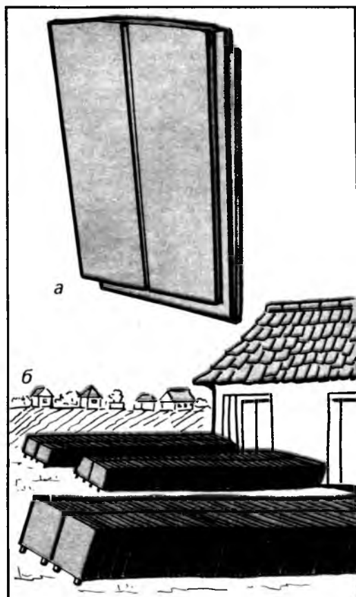
Рис. 5. Готовая черепица: а — из цемента марки 400 и песка средней крупности; б — складирование перед отправкой черепицы
