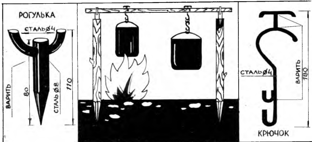
Рис. 5. Комплект принадлежностей для костра
