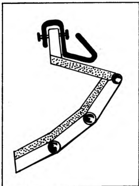
Рис. 3. Установка держателя
