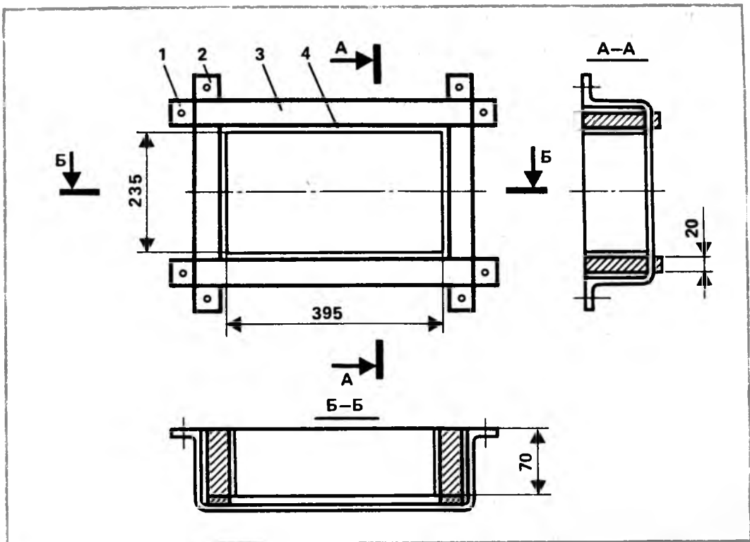
Рис. 3. Форма: 1, 2 — металлические полосы; 3 — стенка; 4 — металлическая окантовка
