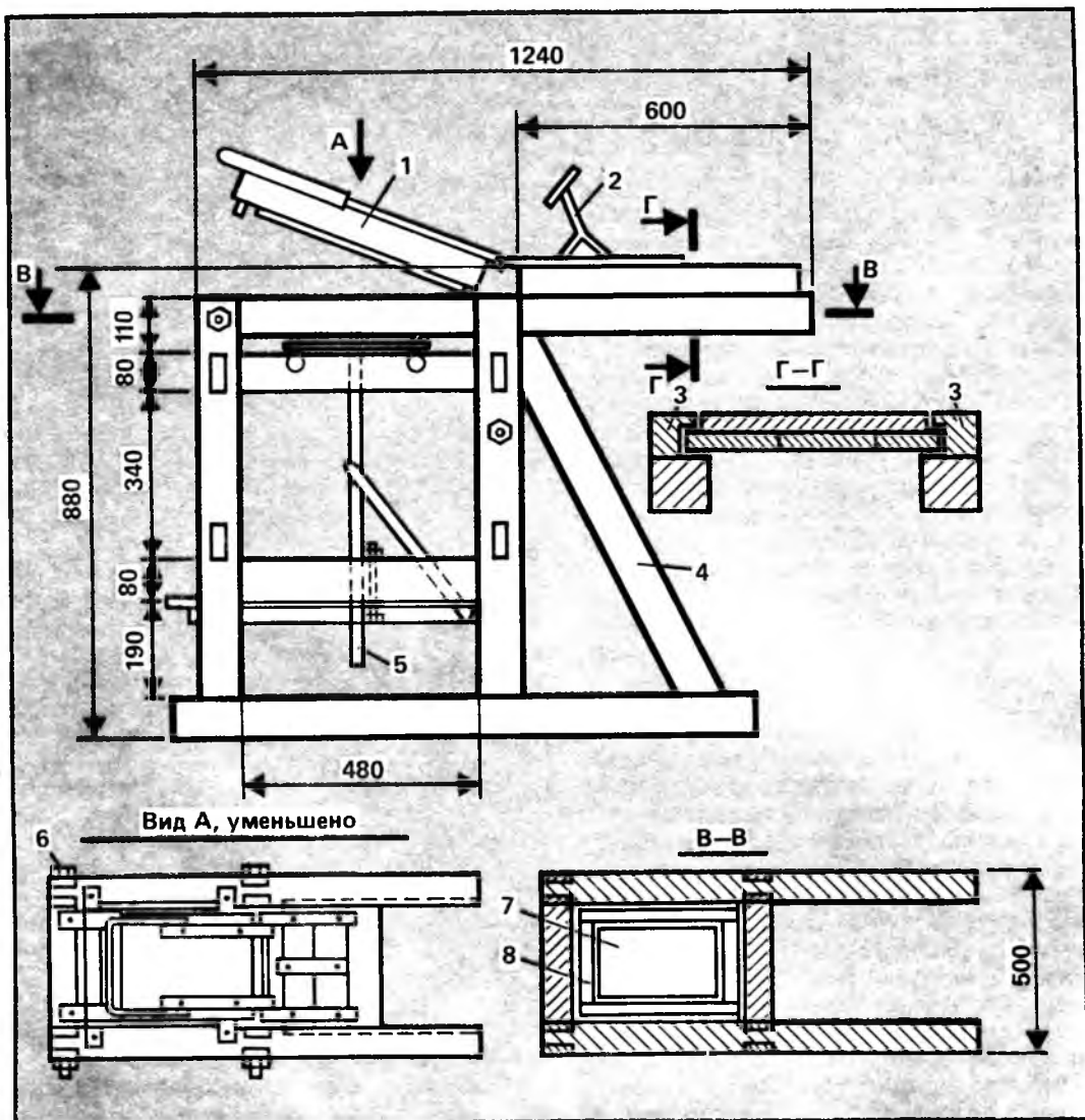
Рис.1. Деревянный формовочный станок: 1 — пуансон; 2 — опора; 3 — брус-ограничитель; 4 — станина; 5 — выталкивающий механизм; 6 — стяжная шпилька; 7 — матрица; 8 — форма
