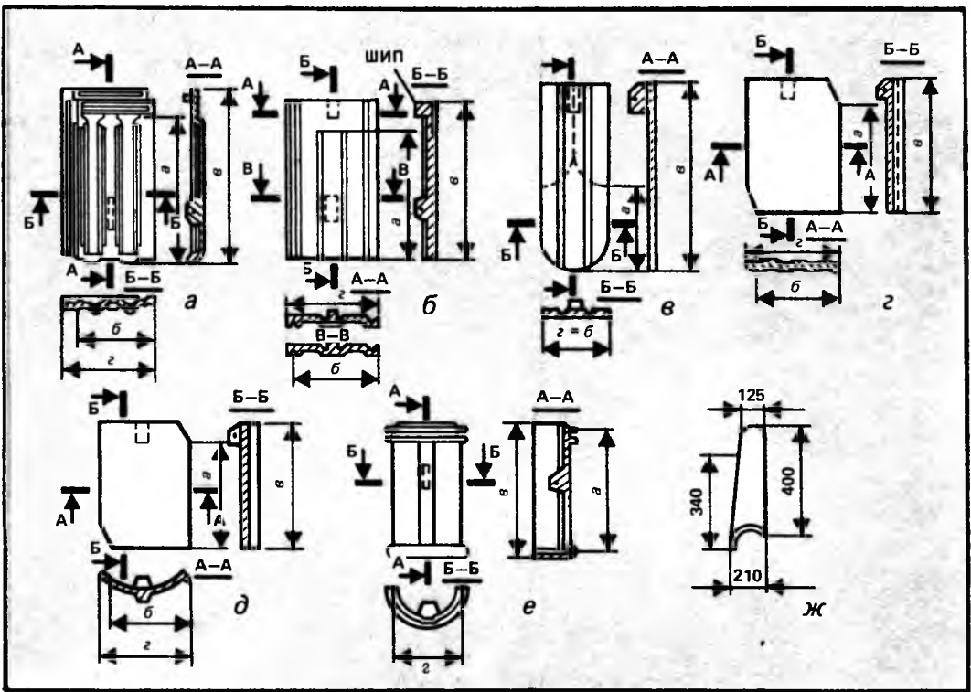
Рис. 9. Глиняная и цементнопесчаная черепица: а — пазовая штампованная; б — пазовая ленточная; в — плоская ленточная; г — волнистая ленточная; д — S-образная ленточная; е — коньковая; ж — желобчатая
