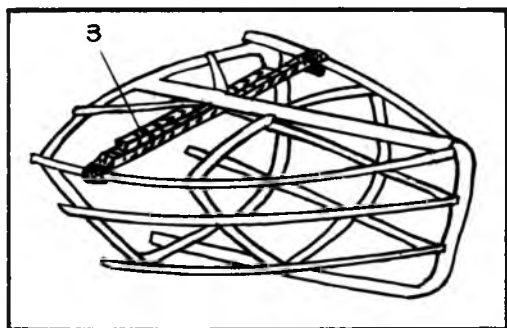
Рис.1. Оборудование кормового сиденья байдарки: 1 — дерево; 2 — скоба (дюралюминий толщиной 2 мм); 3 — кормовой бимс
