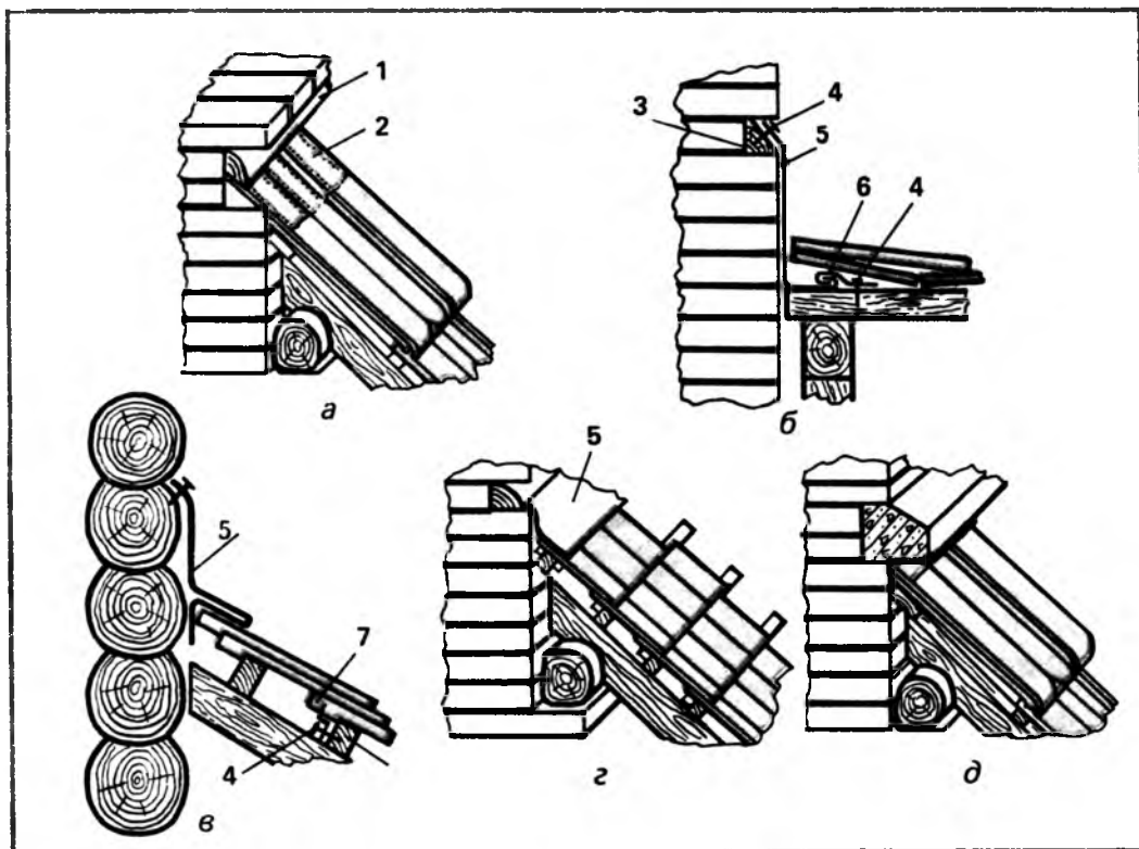
Рис. 19. Премыкание черепичной кровли к вертикальной стене: а — когда в кладке оставлена полость; б — когда в кладку введена закладная рейка; в — когда имеется бревенчатая стена; г — когда в кладку заложен и замоноличен фартук; д — когда в стене козырек; 1 — раствор; 2 — пазовая штампованная черепица; 3 — закладная рейка; 4 — гвоздь; 5 — фартук; 6 — кляммера; 7 — шип плоской черепицы; 8 — брусок
