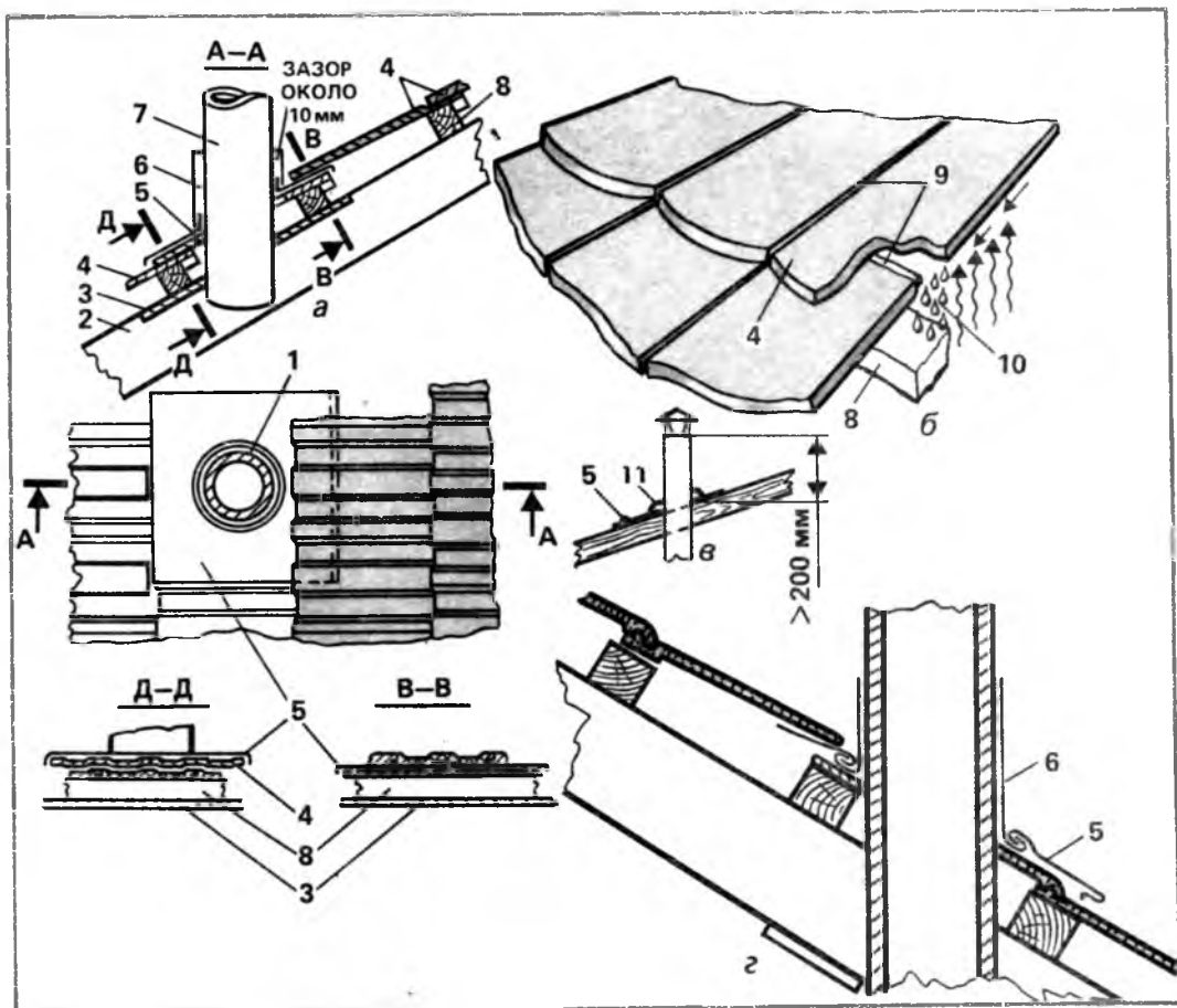
Рис.13. Вентиляция чердака: а — тугое прокрашенное соединение обоймы и воротника; б — промазка швов раствором; в — прокладка или проклейка стыка воротника и обоймы; г — соединение обоймы и воротника одинарным лежащим фальцем; 1 — уплотнение; 2 — стропило; 3 — доска-фиксатор; 4 — черепица; 5 — обойма; 6 — воротник; 7 — вентиляционная труба; 8 — брусок обрешетки; 9 — раствор; 10 — конденсация паров; 11 — прокладка
