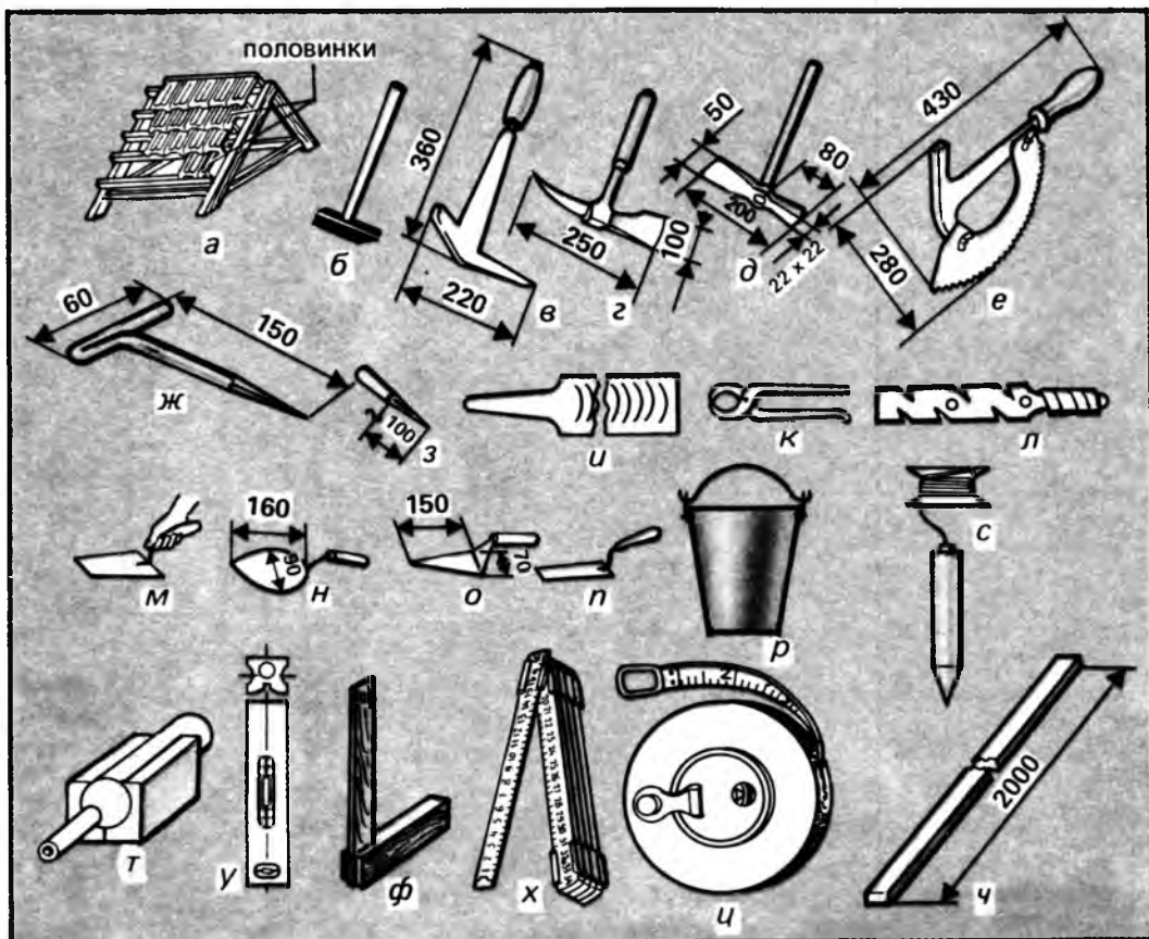
Рис.10. Инструмент и приспособления для покрытия крыши черепицей: а — контрольная обрешетка; б,в — молотки; г — кирочка-топорик; д — кирочка-молоток; е — молоток-ножовка-топорик; ж — развертка; з — трехгранное шило; и — рашпиль; к — клещи; л — гвоздодер; м,н,о,п — кельмы; р — ведро; с — отвес; т — самодельный уровень; у — заводской уровень; ф — деревянный угольник; х — метр складной; ц — рулетка; ч — рейка
