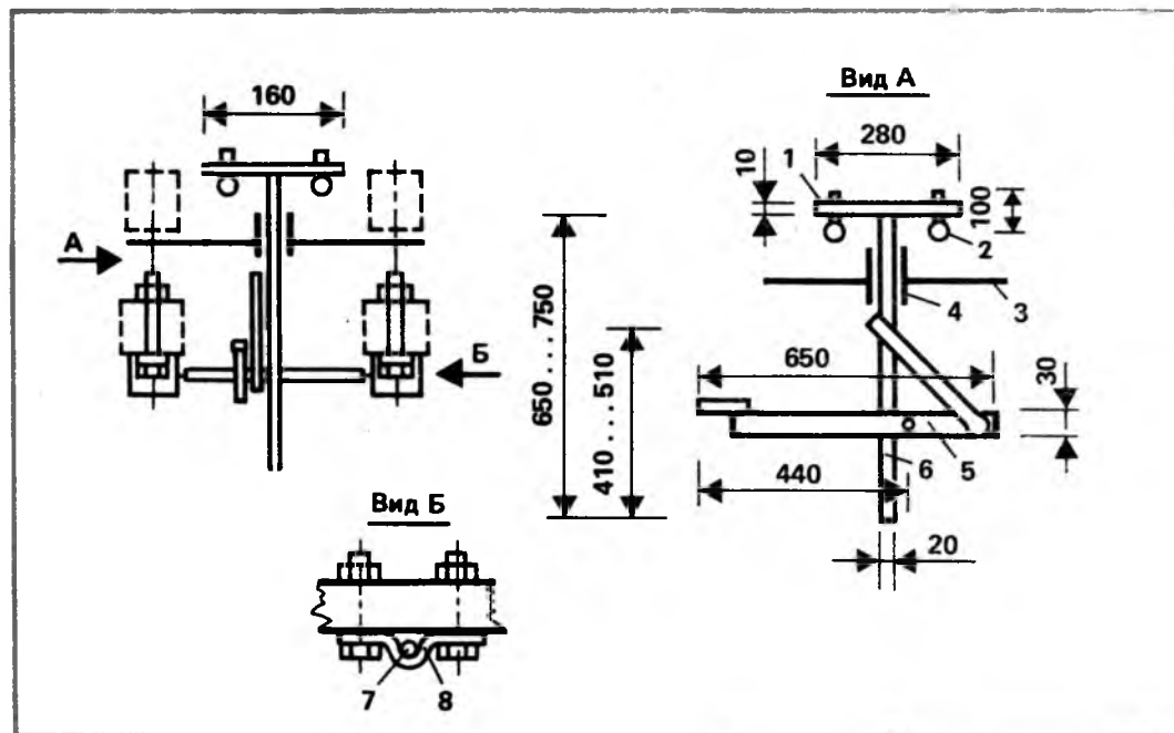
Рис. 4. Выталкивающий механизм: 1 — пластина; 2 — палец; 3 — металлический лист; 4 — втулка; 5 — рычаг; 6 — стойка; 7 — ось; 8 — скоба
