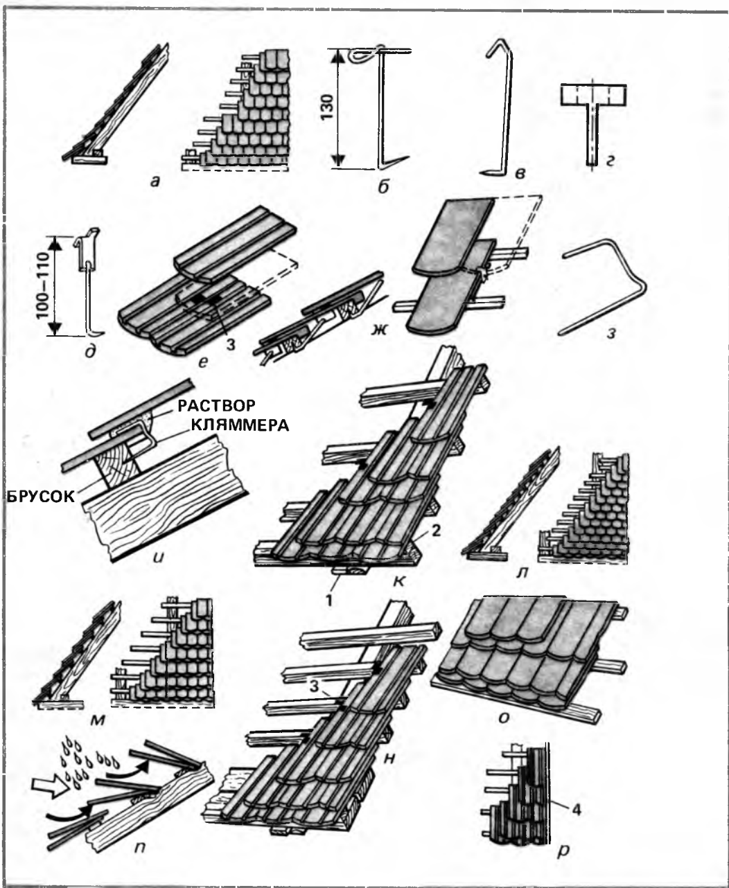
Рис. 14. Укладка плоской ленточной черепицы: а — однослойная; б, в — проволочные кляммеры; г — кляммера из металлического листа; д — комбинированная кляммера; е, ж — установка комбинированных кляммер; з, и — проволочная кляммера и ее установка; к, л — двухслойная укладка черепицы; м — зубчатая укладка; н — чешуйчатая укладка; о — вечноная укладка; п — действие ветра на вечноную укладку; р — стопорение черепицы по фронтонному свесу; 1 — кобылка; 2 — выравнильный брус; 3 — кляммера; 4 — ветровая доска
