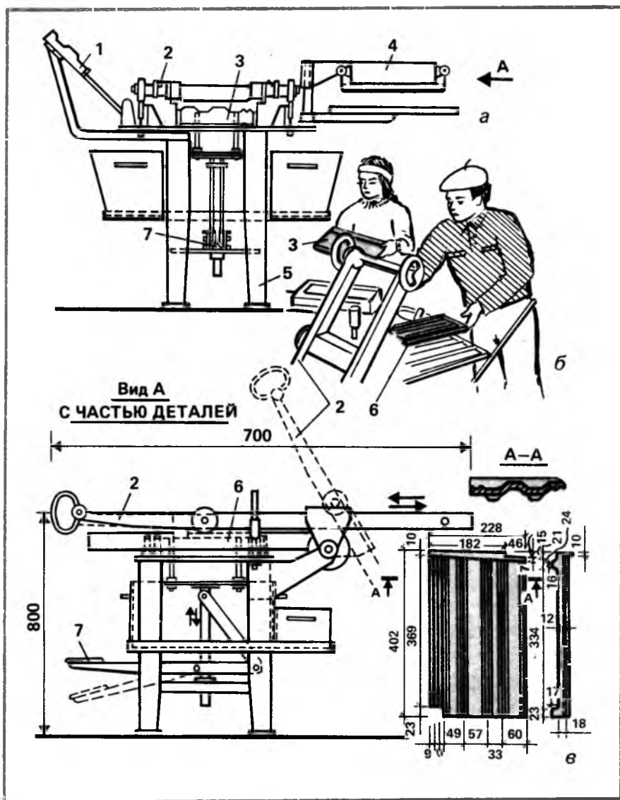
Рис.6. Металлический формовочный станок: 1 — ящик-обрезчик; 2 — каретка-пуансон; 3 — матрица; 4 — ящик с ситом для цемента с красителем или без него; 5 — станина; 6 — форма; 7 — выталкивающий механизм; а — станок; б — работа на станке; в — черепица
